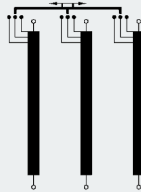
Sternschaltstellung für Transformator Setting for star-connected transformer
