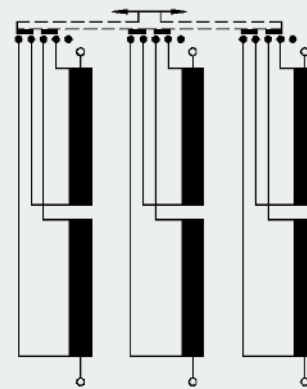
Serien-Parallelschaltung Series-parallel coupling
