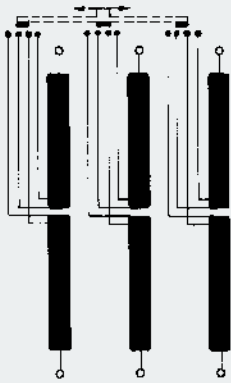
Dreieckschaltung für Transformator Setting for delta transformer
