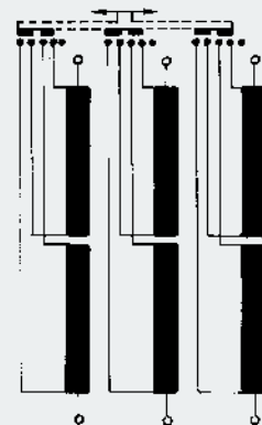
Serien-Parallelschaltung Series-parallel coupling
