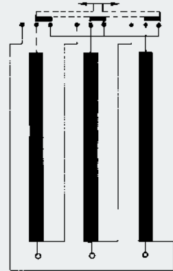
Stern-Dreieckschaltung Star-delta coupling
